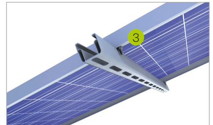
Modulnedglidningssikring monteret i rammebo- ringen
