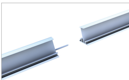
Asetuskiskojen liitäntä profilipeltikatolla
