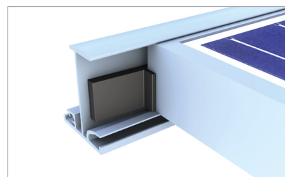
Paneelin varmistus katon kaltevuuden ollessa pieni
