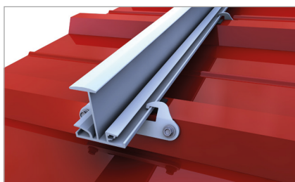
Asetuskisko EPDM-tiivisteellä ja profiiliilitin
