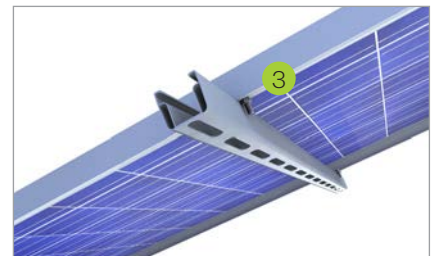
Afglijdbeveiligingsset voor zonnepanelen aan het frameboorgat
