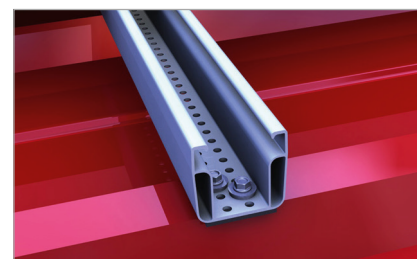
Шаблон за пробиване за къс профил за вертикален монтаж
