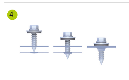
Завинтване без обтягане за по-големи сили на теглене
