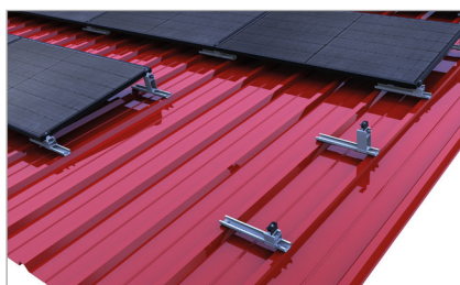
Variant med liggende, standermonterede moduler
