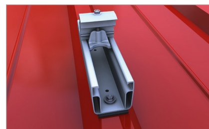
Päättyliitin lyhyessä profilissa C47
