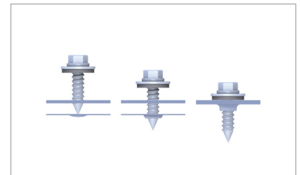
Lastuamaton ruuvikiinnitys varmistaa korkeamman vetokuormankeston
