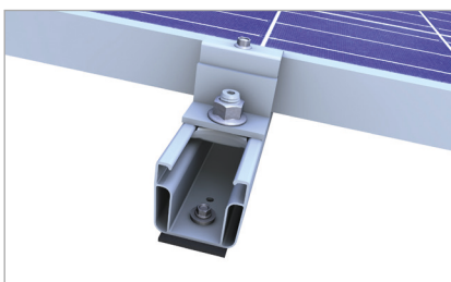
Varmistus lyhyelle profilille tehtävässä vaaka-asennuksessa
