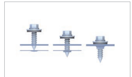
Niet-verspanend vastschroeven voor hogere uittrekrachten
