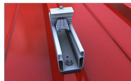
Endeklemme til kortprofil C47
