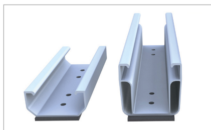
Kortprofiler C24 og C47 til liggende modulmontering
