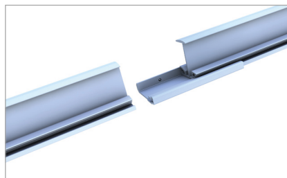
Asetuskiskon kiskoliitin
