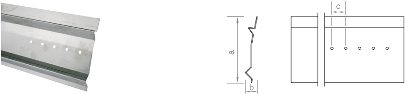
Querträger zur Lastumlagerung, befestigt an den Modulstützen des Flachdachsystems III.
