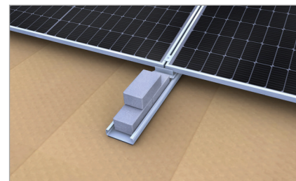
Optionaler Ballastausleger am Anlagenrand
