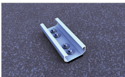
Krátký profil C24 se čtyřmi šrouby pro velké zatížení větrem
