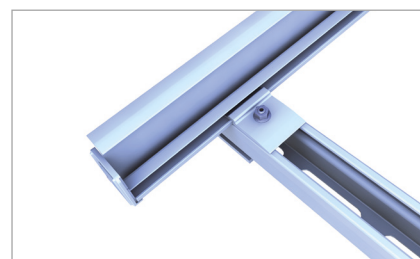
Asetuskiskon kiinnitys C-kiskoon
