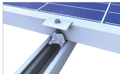
Keskiliitin C-kiskossa 47
