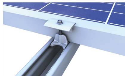
Morsetto centrale nel binario a C 47
